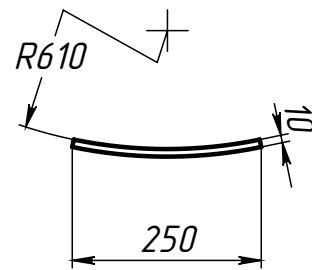
Поз.2 (Ложемент)
