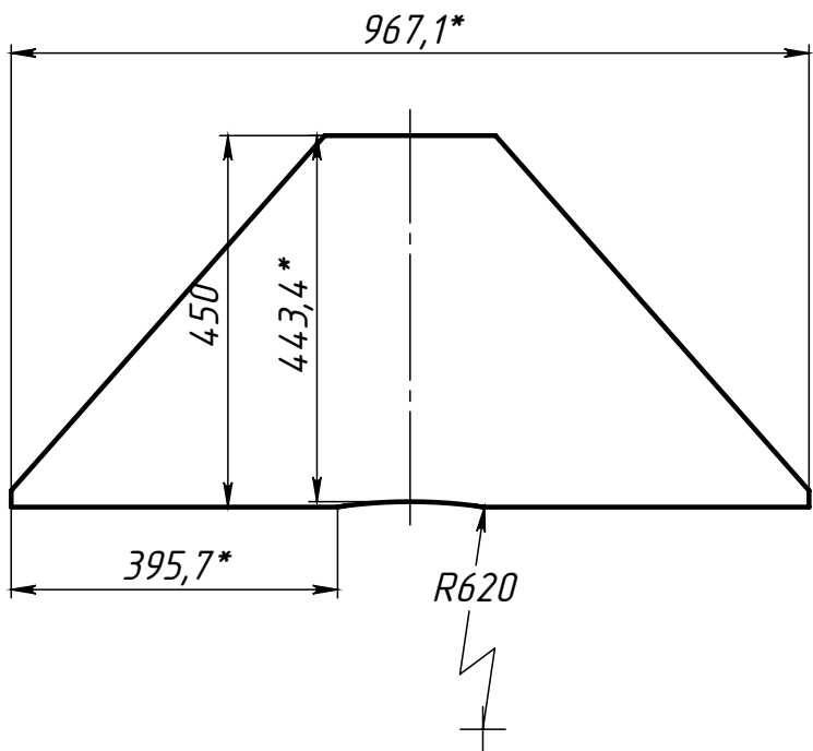
Поз.1 (Корпус) развертка
